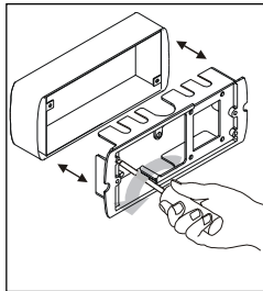
Afb. 2c: Verwijderen van montageframe
