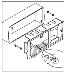
شكل 2c: إزالة هيكل التثبيت
