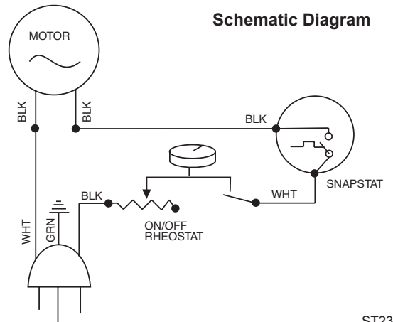
Fig. 43 Fan circuit.
