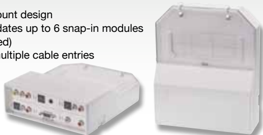
Modular AV & Data Face Plate Box Part No. 60549
