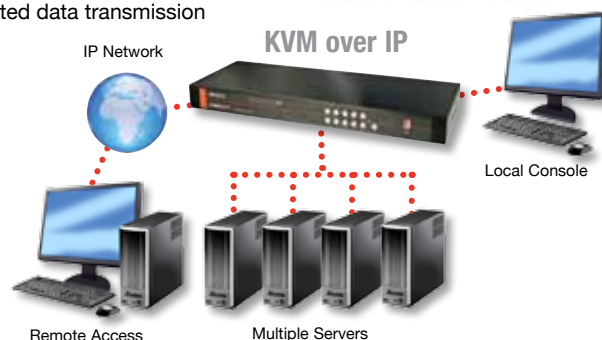
KVM Switch U8
