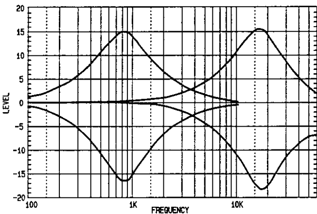
Parametric EQ (HI MID: 1KHz - 16KHz)
