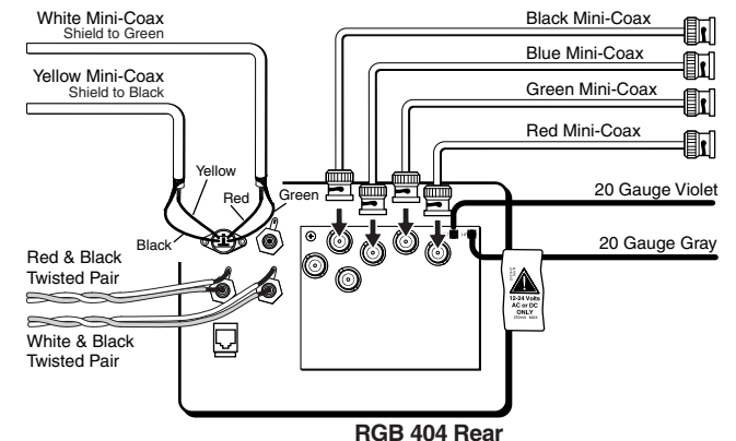
17-Conductor Install Plenum Cable
