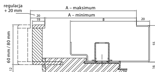
przekrój ościeżnicy PROJEKT Premium
